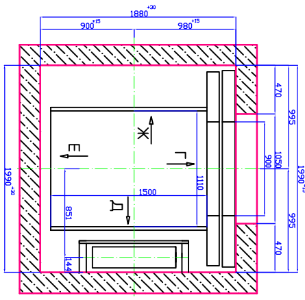
План шахты (повернуто)
