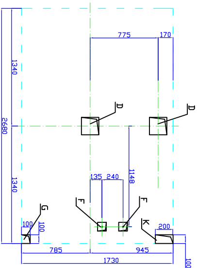
План отверстий в плите перекрытия М.П.
